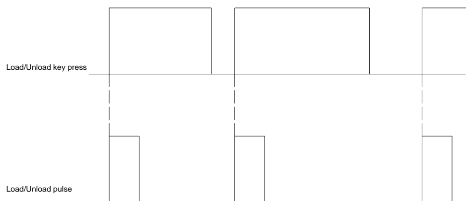
Abbildung 13 – Manuelle Verdichter-Steuerung
