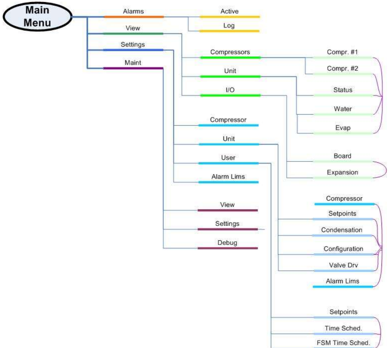
Abbildung 24 - Menüstruktur
