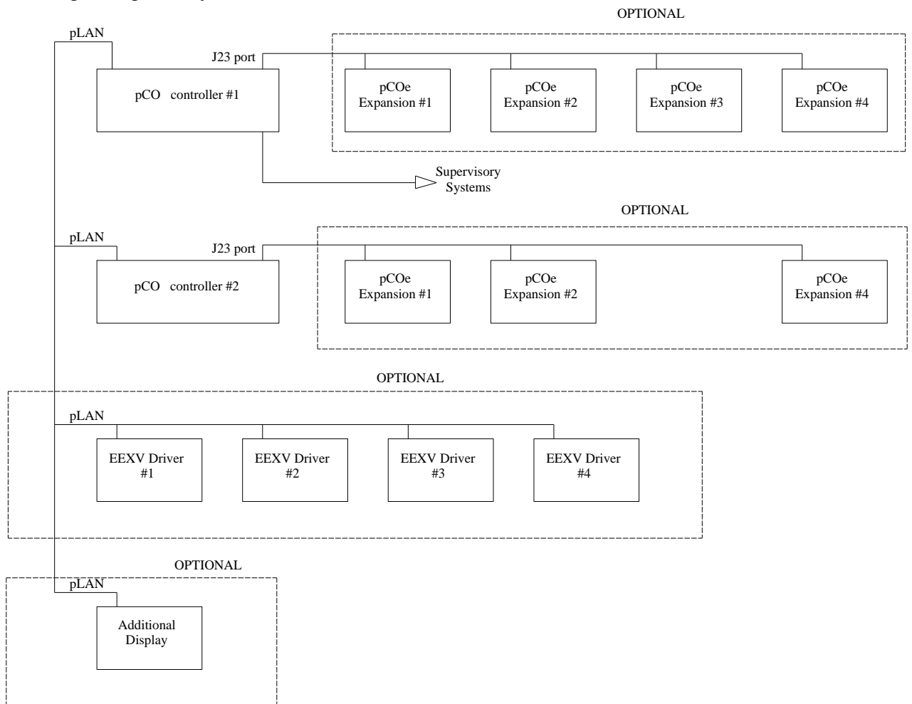
Abbildung 1 – Controller-Architektur
