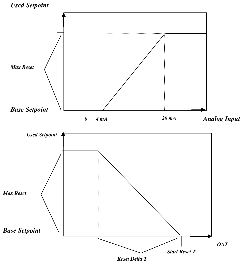
Abbildung 8 - Sollwert-Aufhebung durch 4-20mA-Signale
