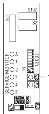
1 Schalter SW3 Fehlerüberprüfung der Verkabelung
