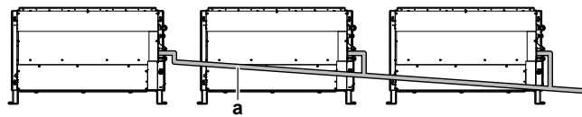
a Zentrales Abflusrohr (mit Gefälle von mindestens 1/100)
