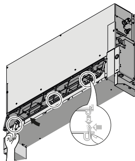
Ansaugen von vorne
