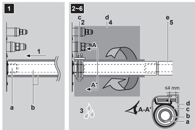
a Abflussrohr-Anschluss (an der Einheit angebracht) b Ablaufschlauch (Zubehör) c Metallschelle (Zubehör)
